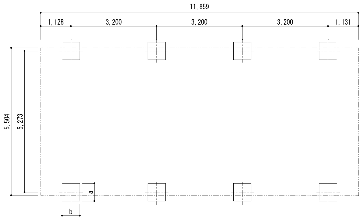
■基礎配置図
